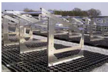
Höhenverstellbare Rahmen und Adapterprofile ermöglichen den Ausgleich von Dachgefälle und die Montage von größeren Modulen.
