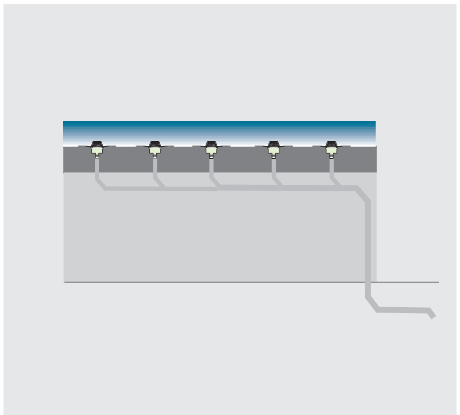
Druckstrom-Dachentwässerung
