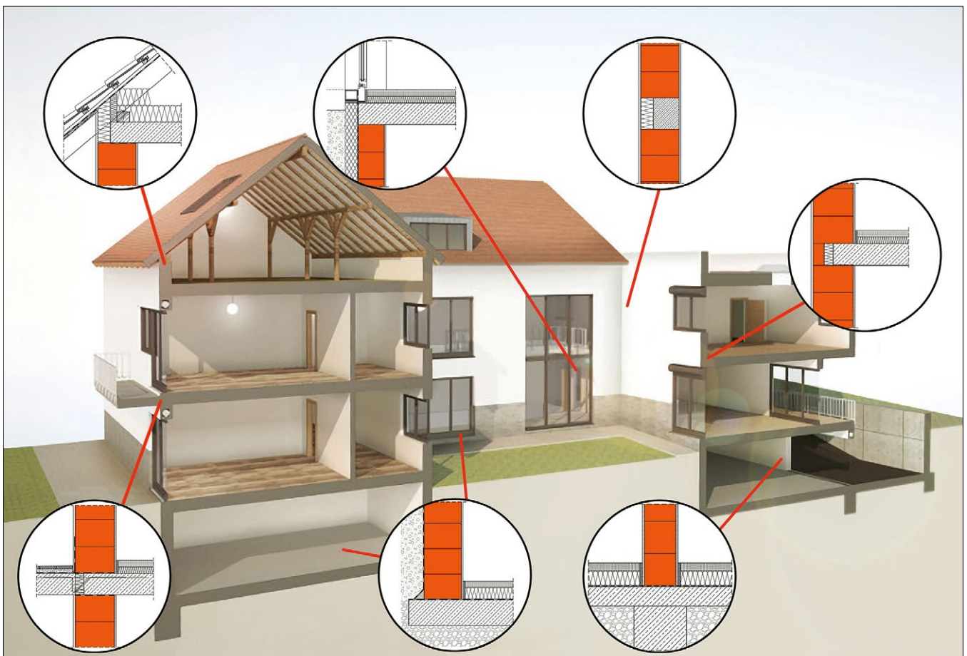
Bild 5.3: Übersicht wichtiger Anschlusssituationen für Wärmebrückendetails im Ziegel Wärmebrückenatolog 5.0
